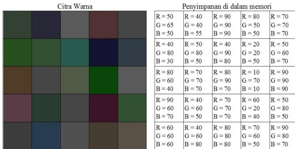
Gambar 2. Penyimpanan citra warna di dalam memori .
