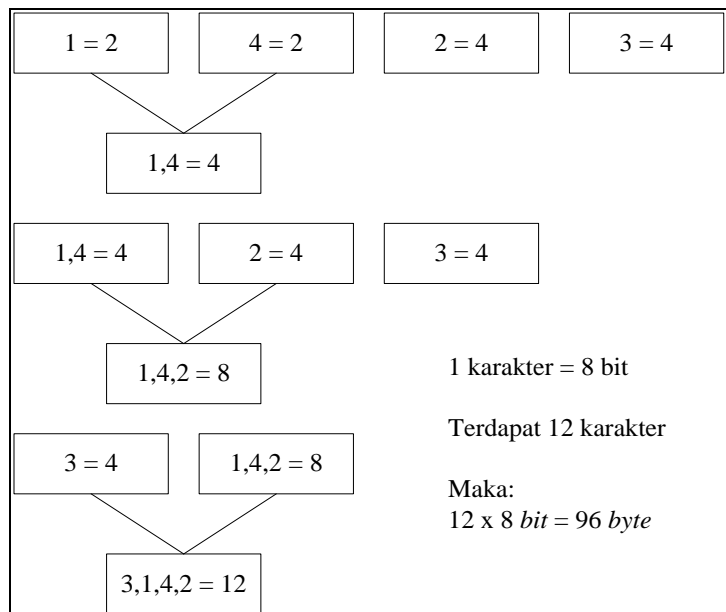
Gambar 9. Pohon huffman sebagai kode huffman
