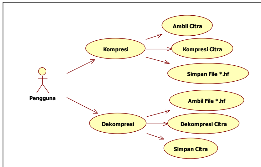
Gambar 11. Use case diagram aplikasi kompresi dan dekompresi
