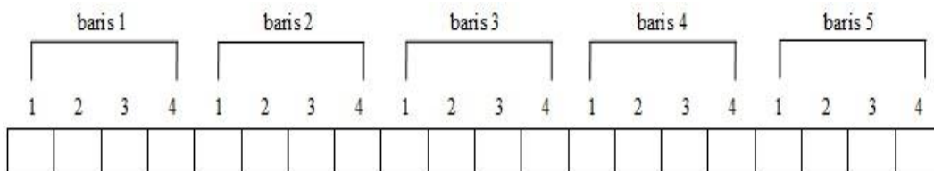
Gambar 4. Representasi matriks 5 x 4 didalam memori sebagai larik
