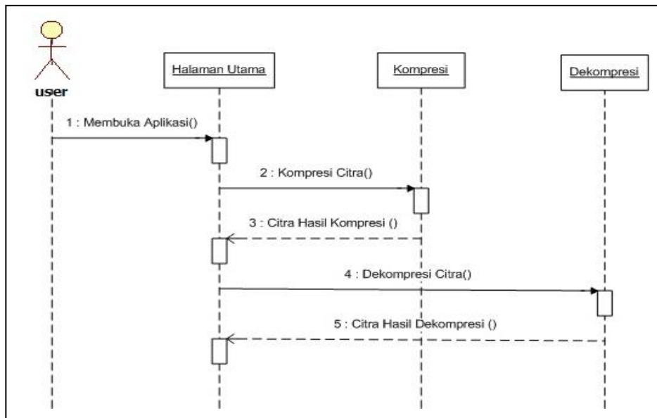
Gambar 13. Sequence diagram rancang bangun applikasi kompresi dan dekompresi
