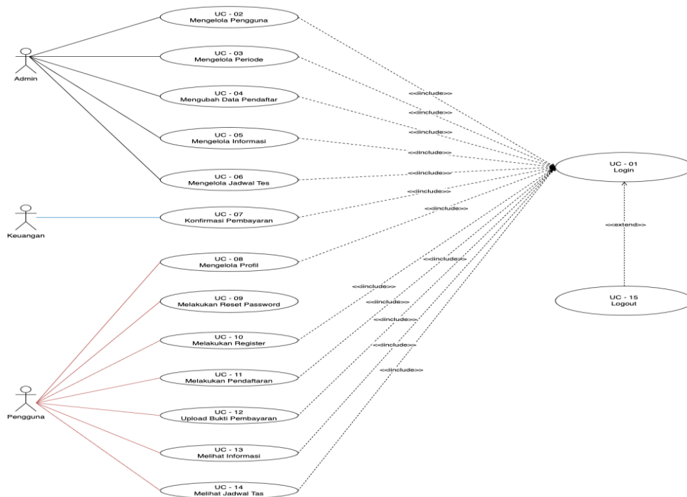
Gambar 3. Use Case Diagram Sistem Penerimaan Santri Baru
