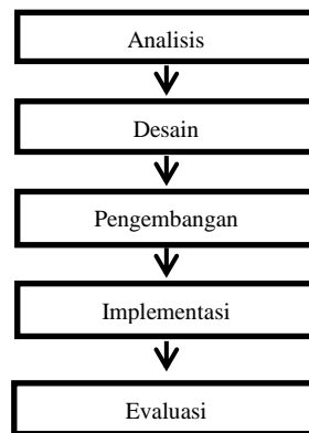
Gambar 1. Tahapan Penelitian
