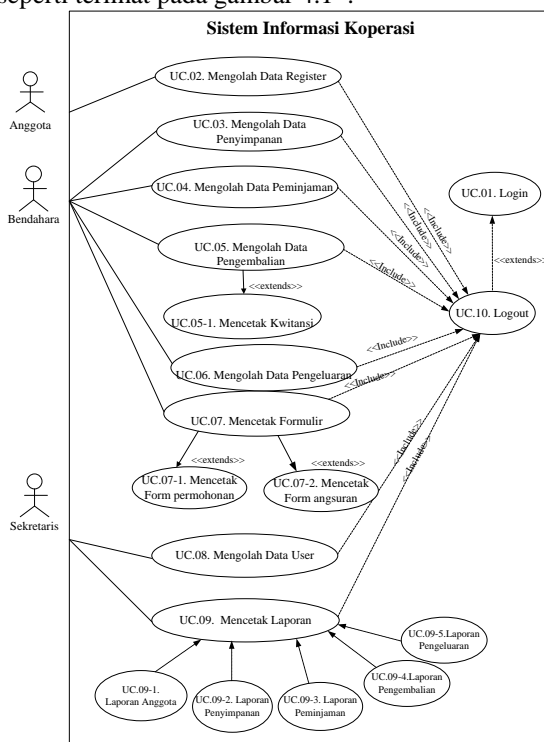
Gambar 4.1 Usecase Diagram Sistem Informasi Koperasi
