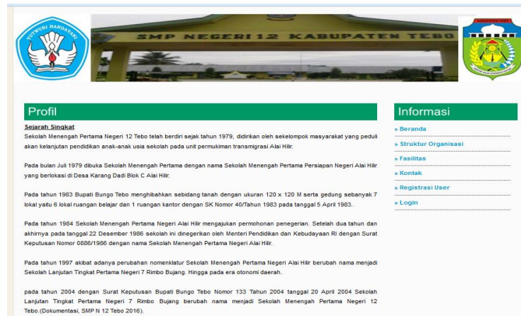
Gambar 4.21 Halaman Awal
