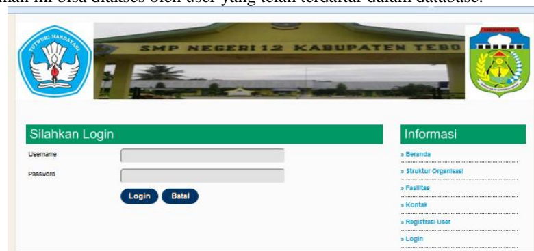
Gambar 4.22 Halaman Login
